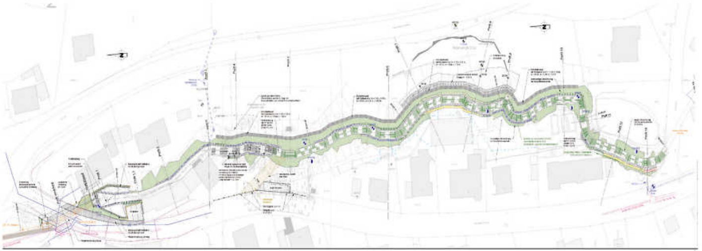
Hochwasserschutz in Sulpach zwischen Seeweg und Sulpacher Straße Pläne: Tractebel GmbH
